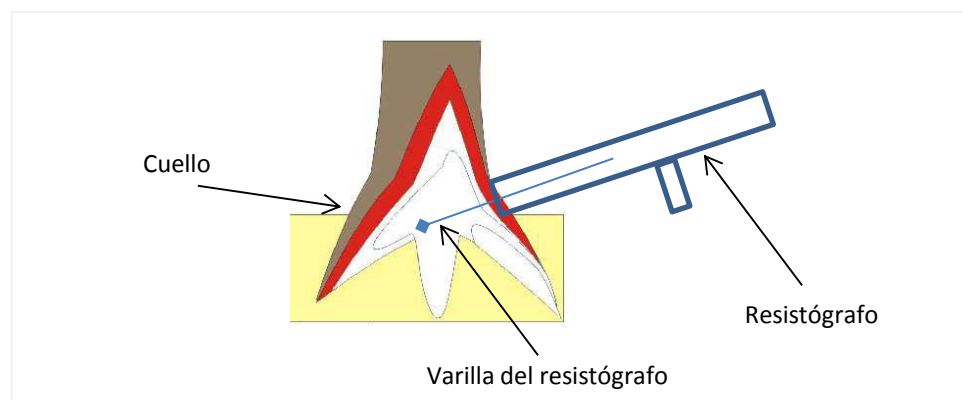
Sistema de detección de pudrición y cavidades internas con resistógrafo
